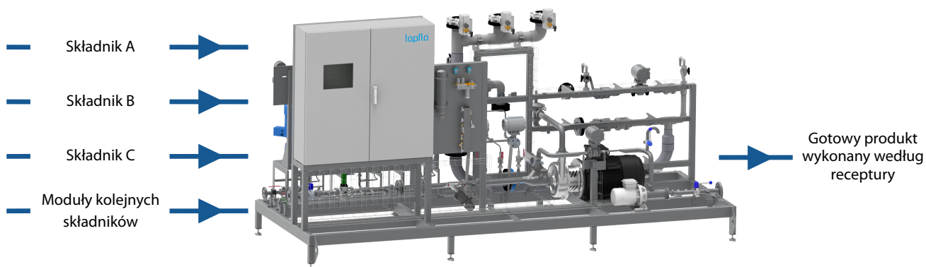
Mieszalnik pracujący w trybie in-line
